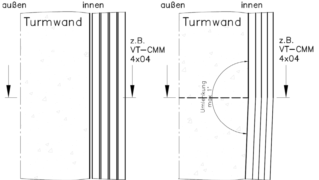
Schnitt VT-CMM 2x04
